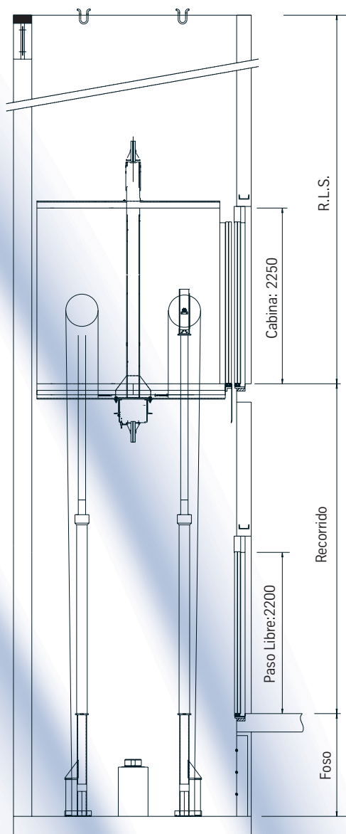
ALZADO
