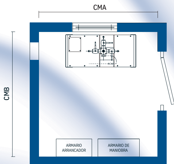
CUARTO DE MÁQUINAS
