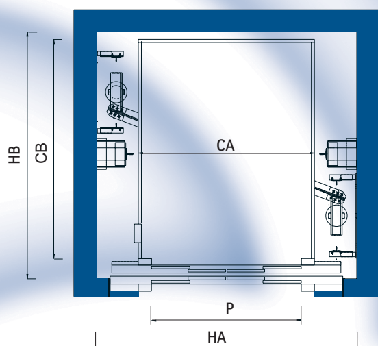
PLANTA DE HUECO
