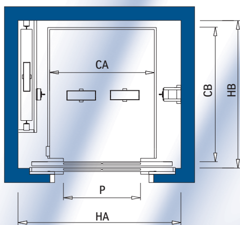
PLANTA DE HUECO
