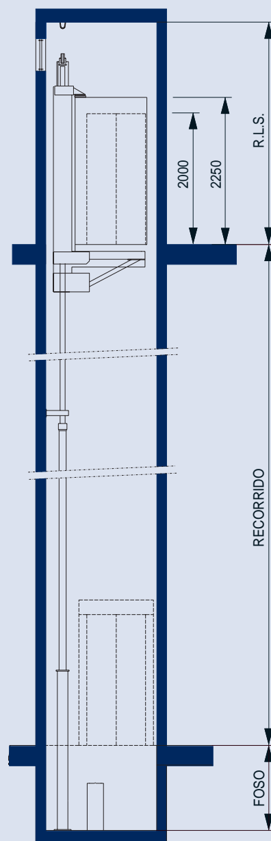
ALZADO
