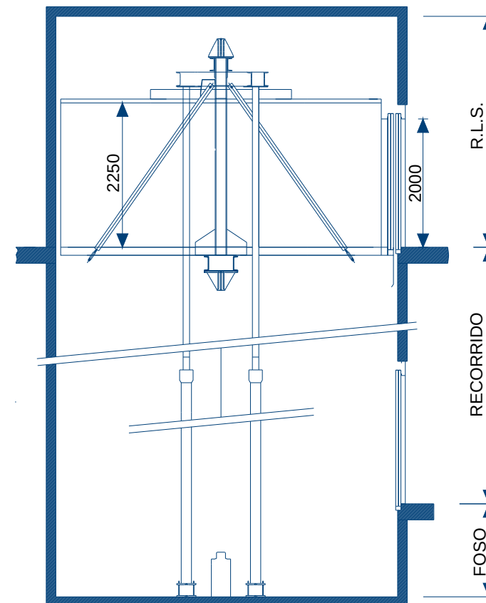
ALZADO
