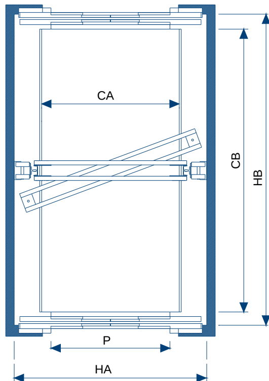
PLANTA DE PISO
