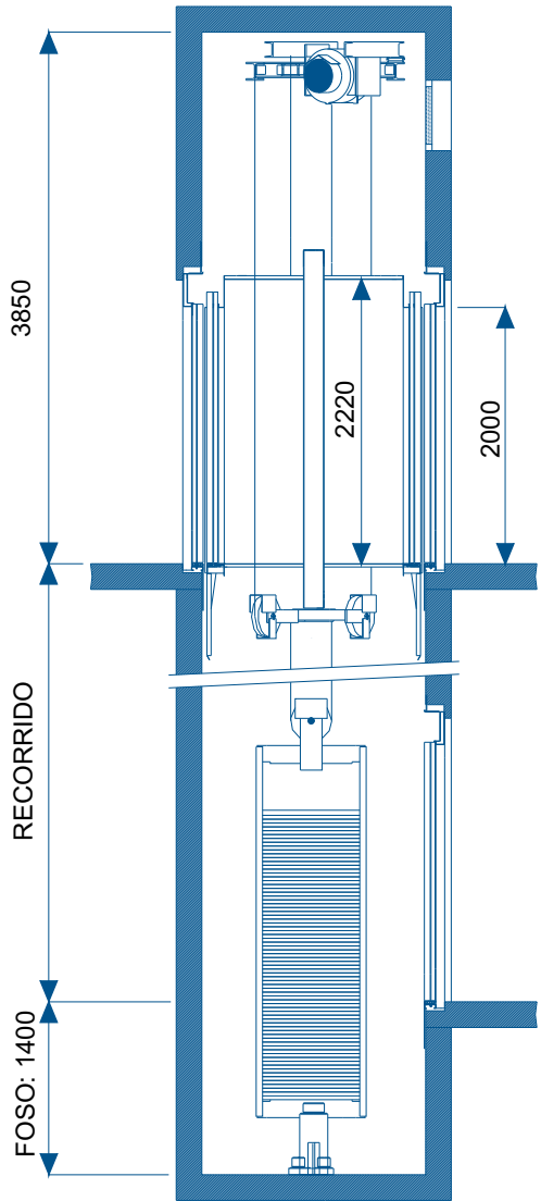
ALZADO
