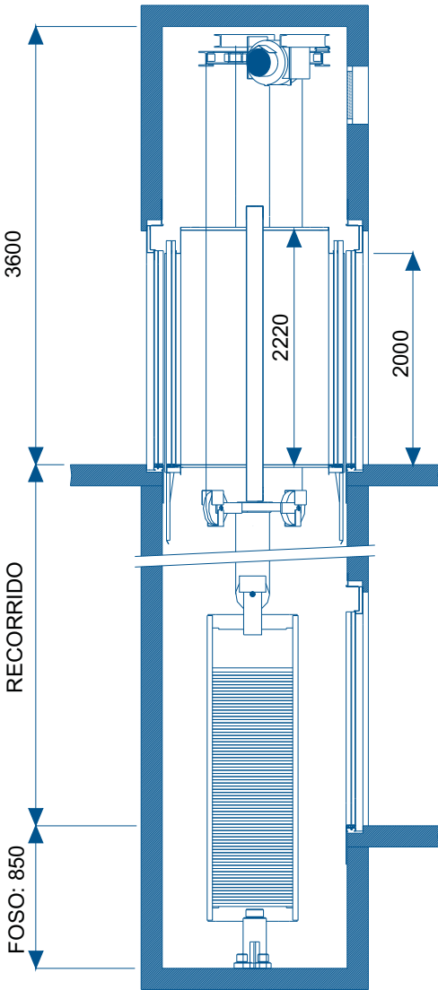
ALZADO
