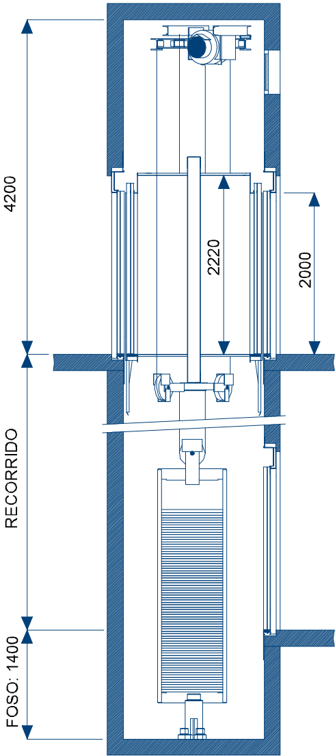
ALZADO
