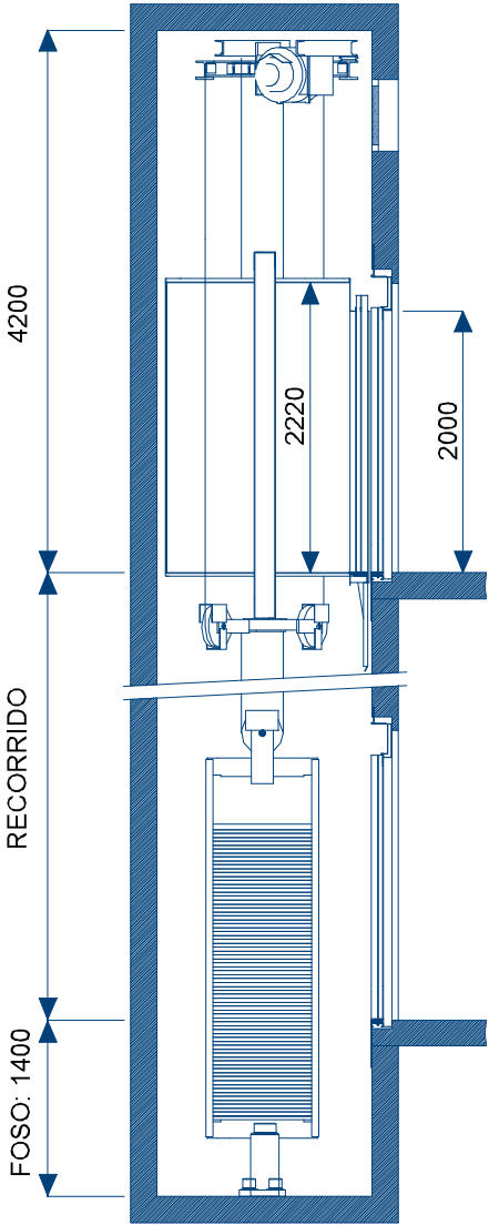
ALZADO
