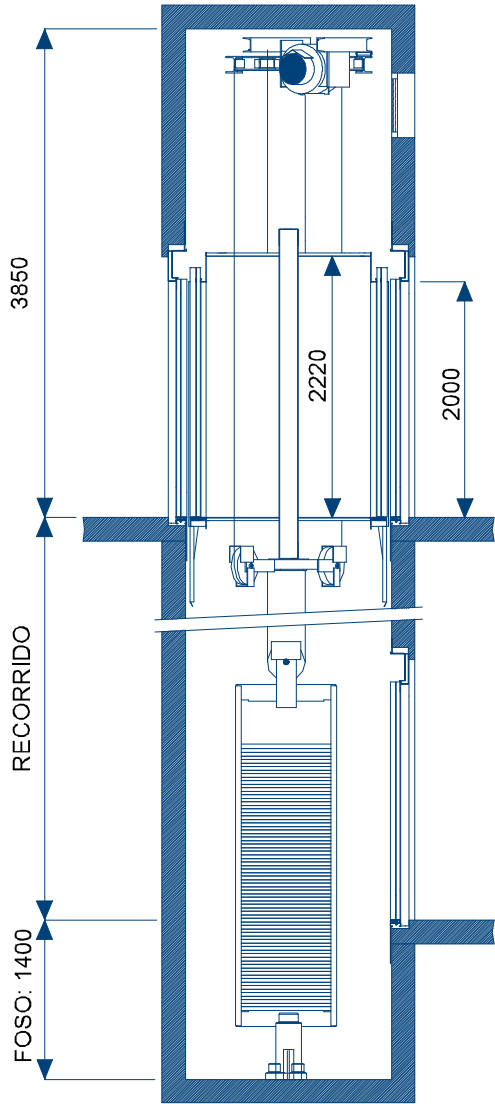
ALZADO
