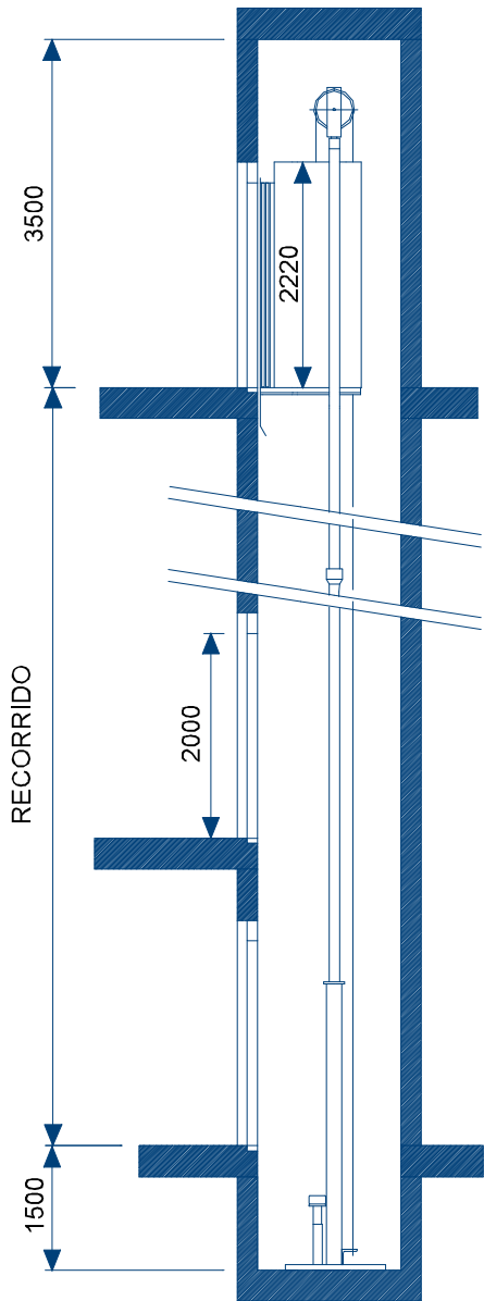
ALZADO
