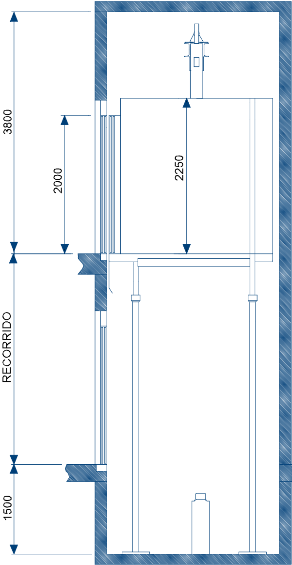
ALZADO
