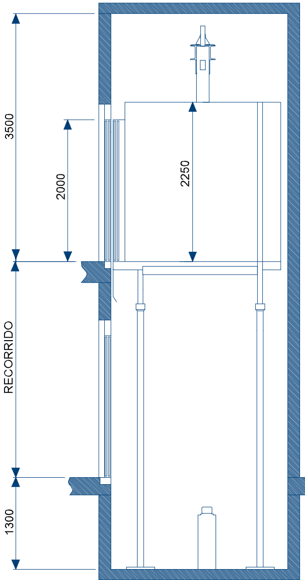
ALZADO
