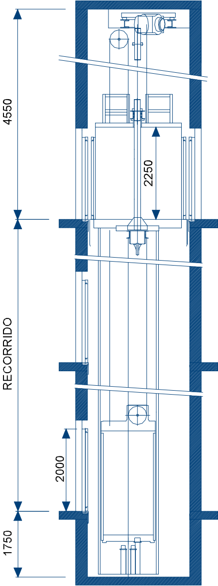
ALZADO
