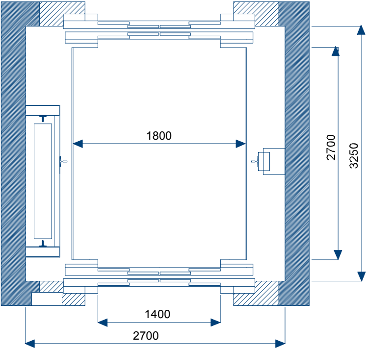
PLANTA DE PISO
