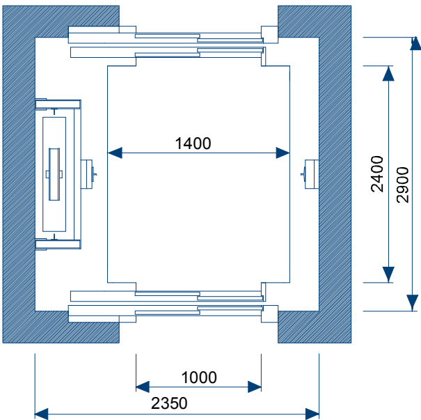
PLANTA DE PISO
