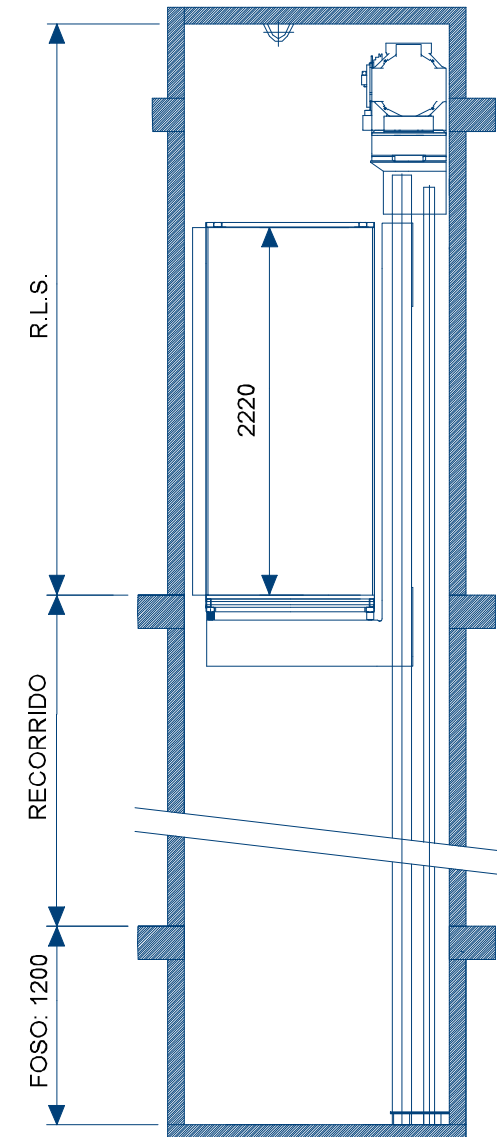
ALZADO
