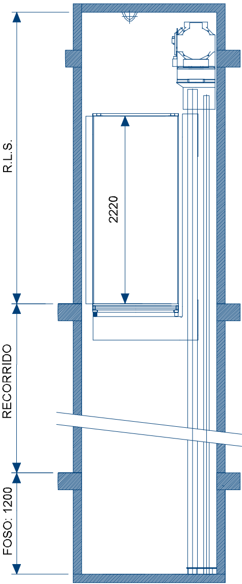
ALZADO
